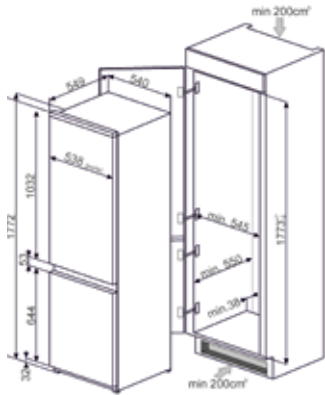
C3170P
