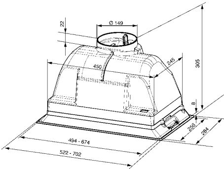
KSEG7XE KSEG5XE
