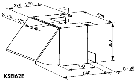
KSEI62E
