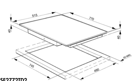
SE2772TD2
