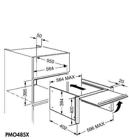
PMO485X
