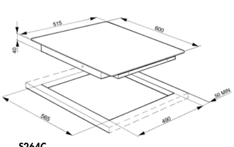
S264C
