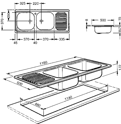
LX116D-2 LX116S-2
