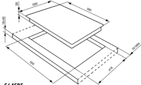
S64SBE
