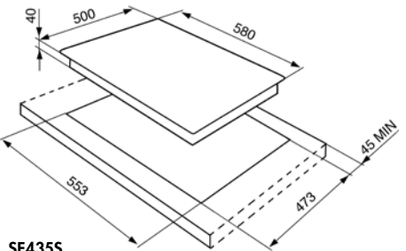
SE435S
