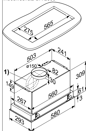
Inbouwschets DA 2660
