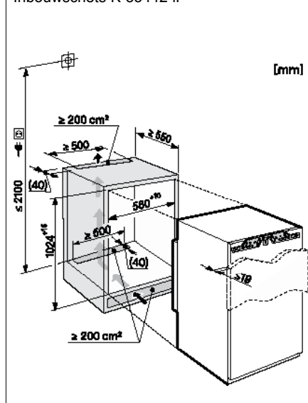
Inbouwschets K 33442 iF
