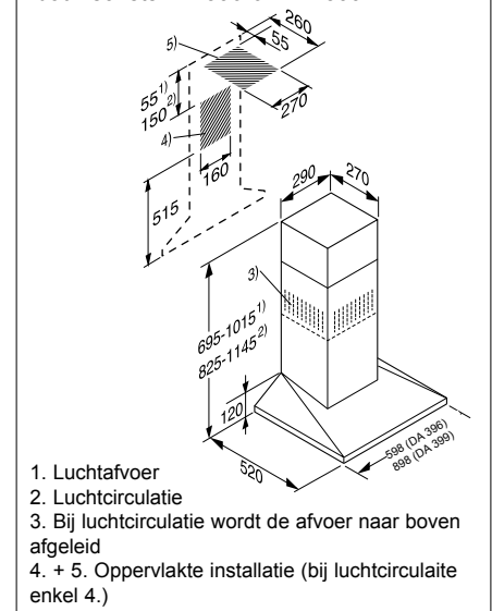
Inbouwschets DA 396-6 / DA 399-7
