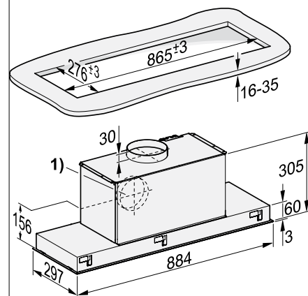
Inbouwschets DA 2390
