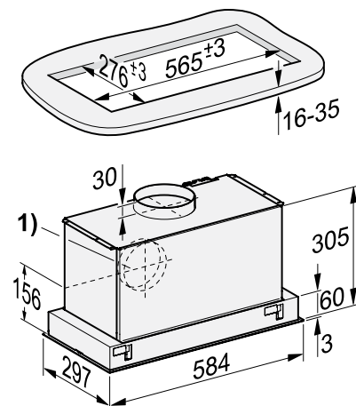
Inbouwschets DA 2360
