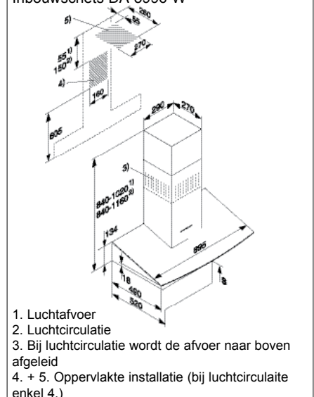
Inbouwschets DA 5996 W
