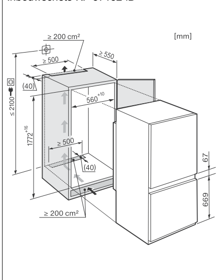
Inbouwschets KF 37132 iD
