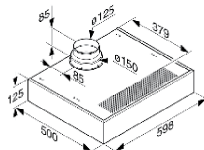
Inbouwschets DA 1260
