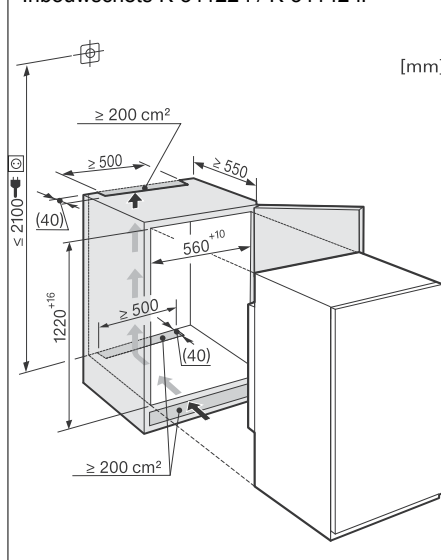
Inbouwschets K 34122 i / K 34142 iF
