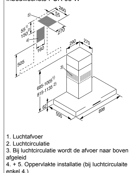
Inbouwschets PUR 98 W
